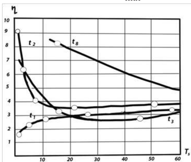
Рис.2. Зависимость показателя \eta от числа информационных k символов при различной корректирующей способности t_i
