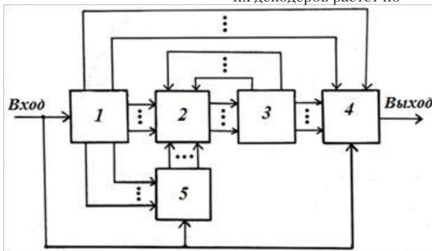
Рис.1. Структурная схема устройства адаптивного мажоритарного декодирования
